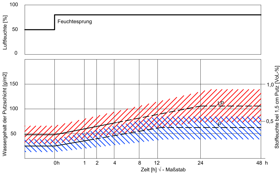
Abb.4 Wasserdampfabsorption von Innenputzen nach Erhöhung der Umgebungsfeuchte von 50 auf 80% r.F. bei 20 °C (Feuchtesprungversuch) Grafische Auswertung der in [15] ermittelten Sorptionswerte von unbehandelten Putzschichten d=15mm LP durchschnittliche Lehmputze, Mittelwert P andere Putze (Kalkzement, Gips, Kalkgips), Mittelwert Durchgezogene Linie: Sorptionsfeuchte im normalen Bereich von 50-65% r.F.
