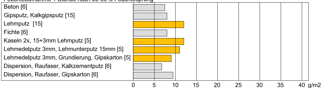
Abb.5 Feuchteaufnahme von Baustoffen und Bauteilen in g/m² nach 1 Stunde nach Feuchtesprung 40-80% und 50-80% r.F. bei 20°C
