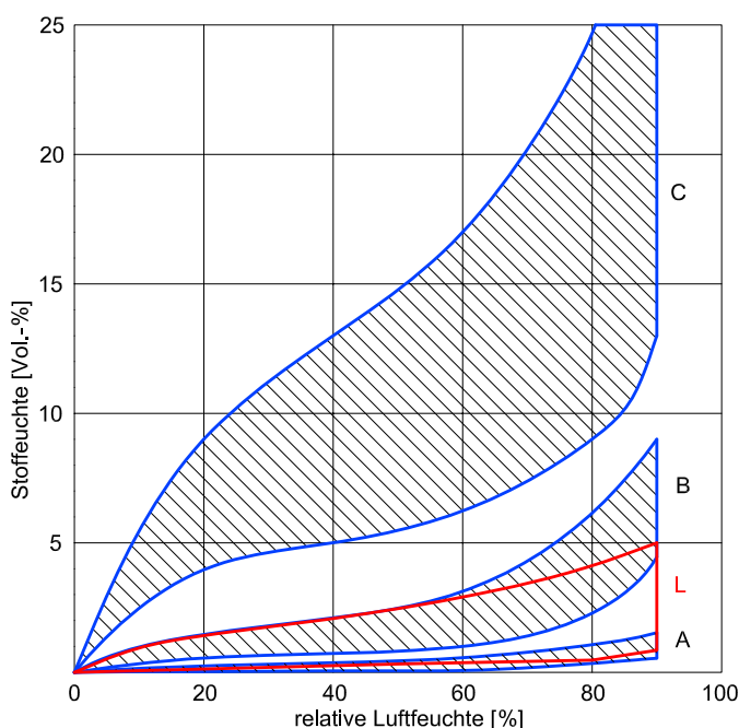
Abb.1 Bereiche der Sorptionsfeuchte von verschiedenen Stoffgruppen in Abhängigkeit von der relativen Luftfeuchte bei 20°C A Ziegel, Gips [8] B Normalbeton, Leichtbeton, Porenbeton, Kalksandstein [8] C Holz, Papier, organische Faserstoffe (Wolle, Seide, Leinen) [8] Anmerkung: L Lehmbaustoffe nach Abb.2 in A einzuordnen: Putze (Lehm, Kalk, Gips) in B teilweise einzuordnen: Sonstige Lehmbaustoffe
