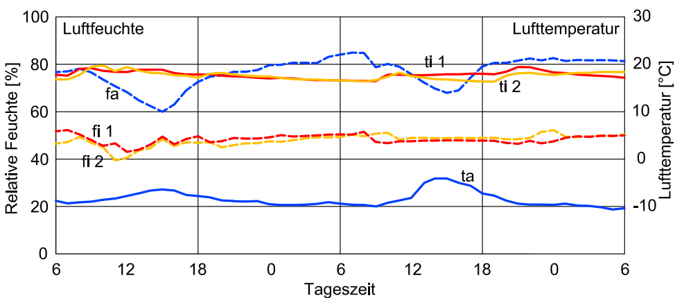
Abb.7 Raumklima im Lehmhaus 1 zwei unterschiedlich verputzte Wohn-Schlafräume einer 2-1/2 Zimmerwohnung Zweipersonenhaushalt, 40m 2 Wohnfläche/Person kalter Januar, tagsüber Luftverbund Wohn-Schlafräum 1: Lehmputz mit Lehmanstrich, 1 Person Wohn-Schlafräum 2: Kalkgipsputz mit Kalkanstrich, 1 Person
