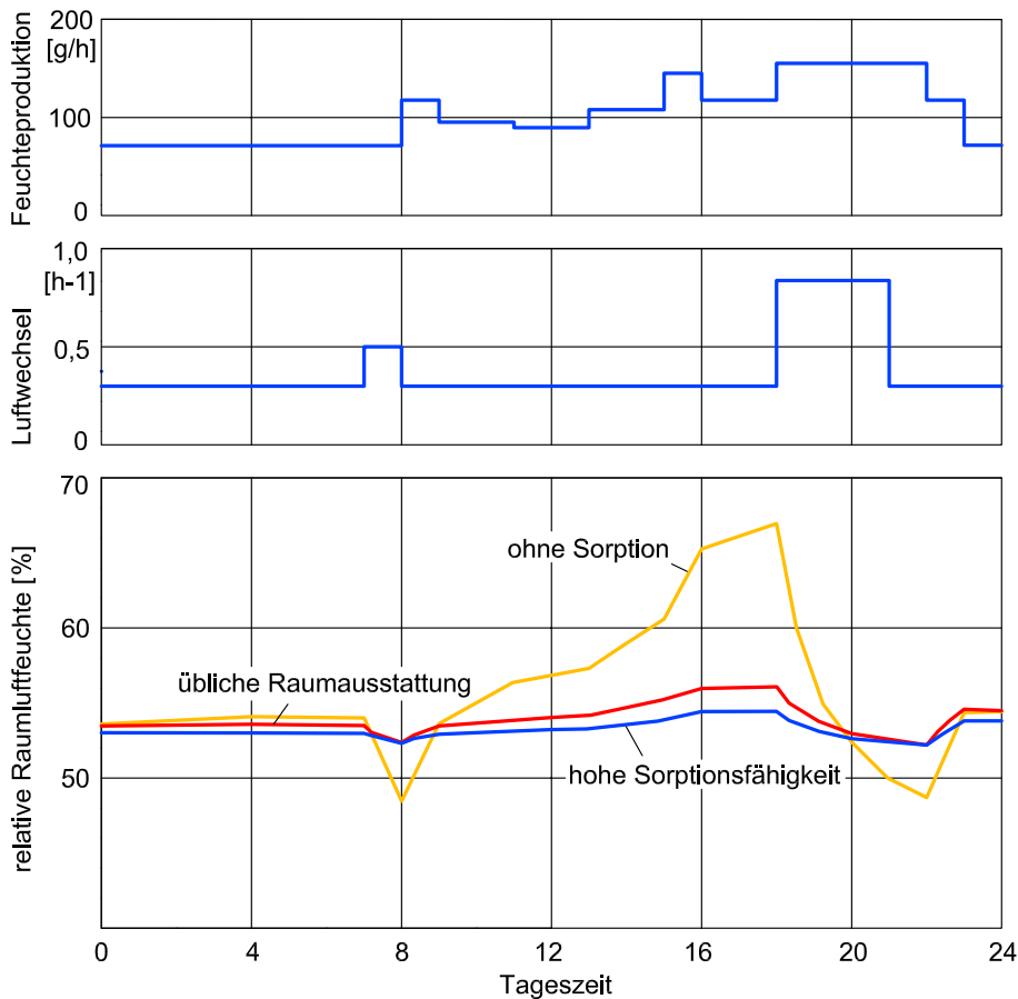
Abb.6 Simulierter Tagesverlauf der Luftfeuchte in einem Wohnzimmer mit unterschiedlicher Sorptionsfähigkeit der Baustoffe und der Ausstattung an einem Wintertag t_{La} = i.M. 0,7 \text{ °C} bei 89% r.F., nach [6][16]
