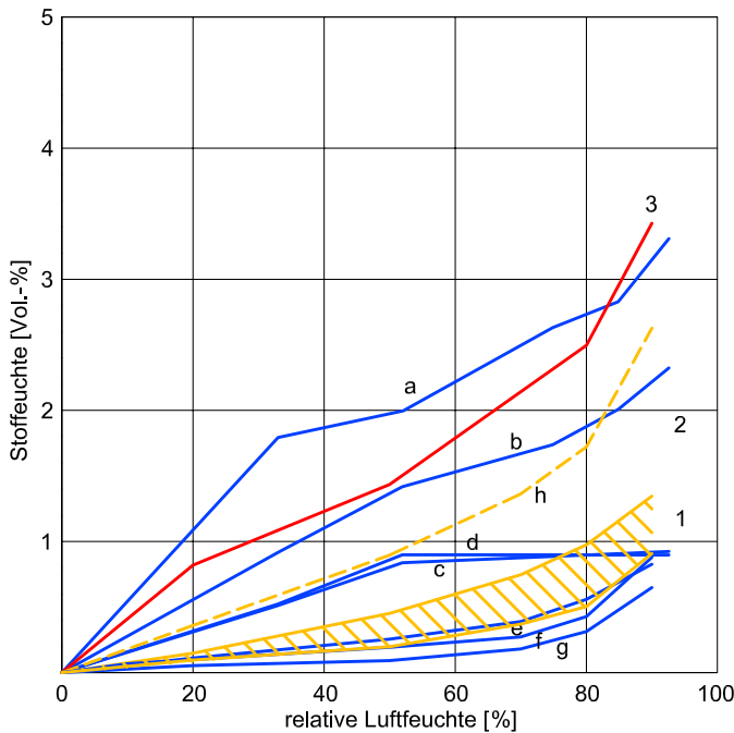
Abb.3 Bereiche der Sorptionsfeuchte von Lehmputzen im Vergleich
