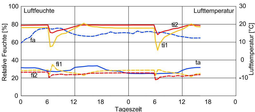
Abb.8 Raumklima im Lehmhaus 2 Atelierraum 1, Bibliothek 2, Luftverbund, nur Tagesnutzung, 1 Person, 120m 2 Wfl/Person, intensive Morgenlüftung, kalter Januar Lehmputz 15mm, Kalkfeinputz 5mm, Kalkanstrich
