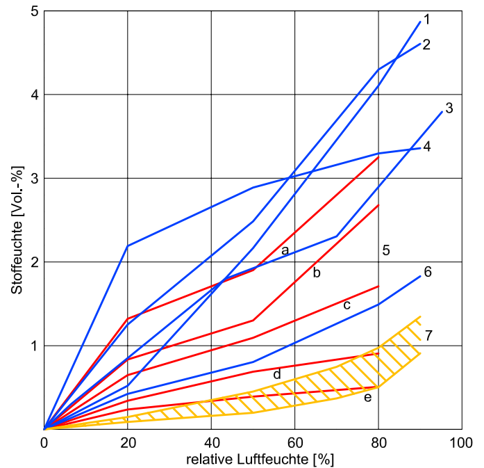
Abb.2 Bereiche der Sorptionsfeuchte von Lehmbaustoffen
